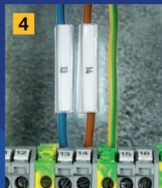
4 Сдвигаемая маркировка
