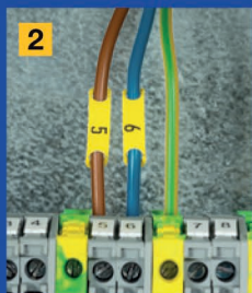
2 Этикетки Rapido
